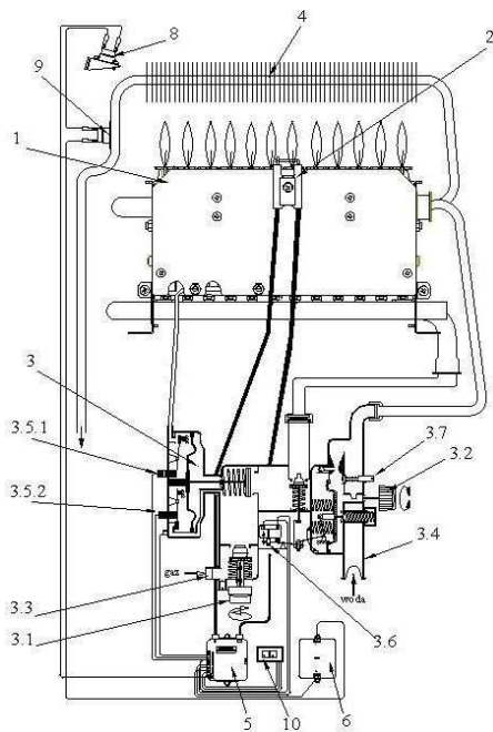
Obrázek 2.2.1.2 Konceptní schéma ohřívače
