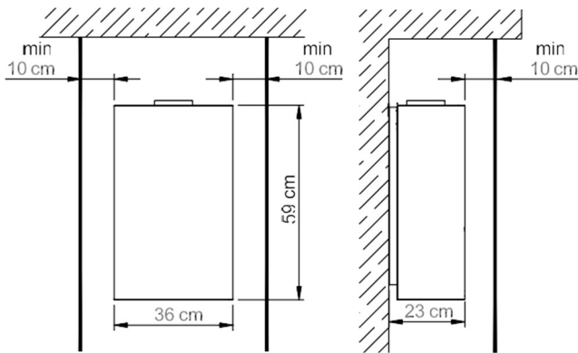
Obrázek 3.3.1 Požadované montážní vzdálenosti
