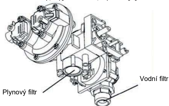
Obrázek 6.4.1 Vodovodní a plynové armatury
