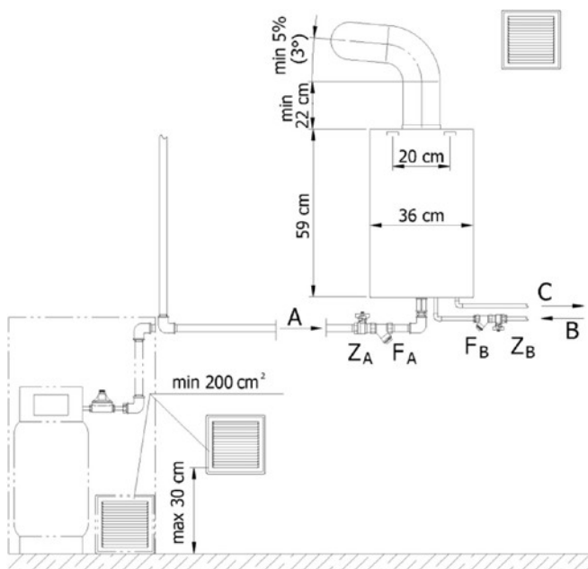
Obrázek 3.1.3.1 Schéma instalace vody, plynu a odvodu spalin
