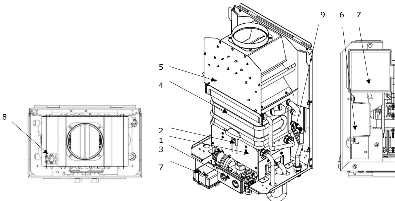
Obrázek 2.2.1.1 Hlavní součásti ohřívačů
