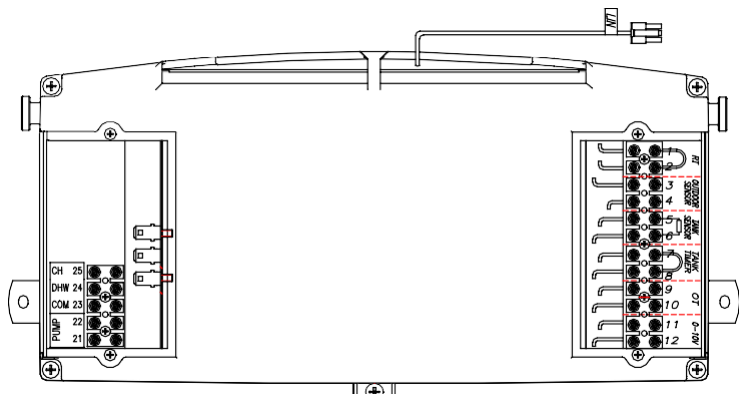
Obrázek 3.9.1.a Elektrické svorky řídicí jednotky pro dvoufunkční kotle
