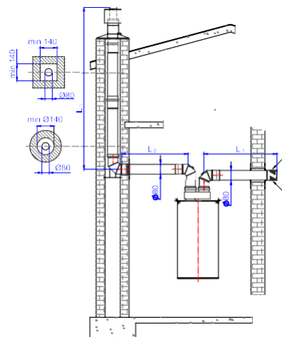
H_{\max} = L_1 + L_2 + L_3 + (1 \text{ m} + 1 \text{ m} + 1 \text{ m}) \text{ (ztráta na kolenech)} Obrázek 3.8.3.2
