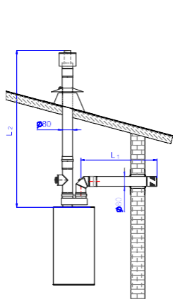
H = L_1 + L_2 + 1 \text{ m (ztráta na kolenu)} Obrázek 3.8.3.1
