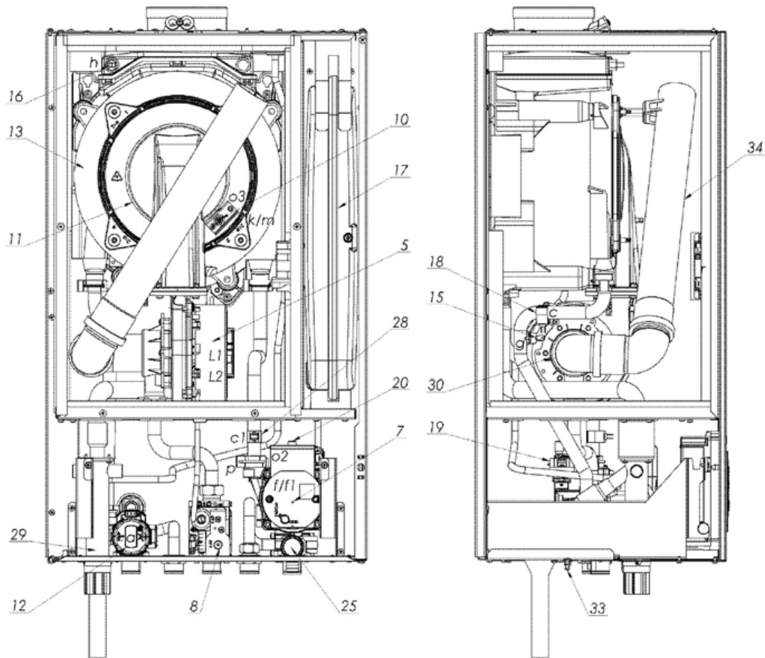
Obrázek 2.2.1.2 Uspořádání součástí v jednofunkčním kotli Ecocondens Nex
