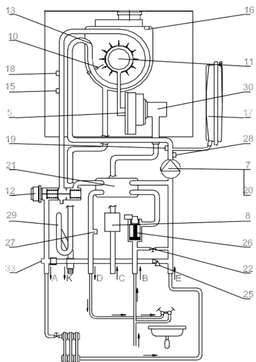
Obrázek 2.2.1.2 Uspořádání součástí v jednofunkčním kotli Ecocondens Nex
