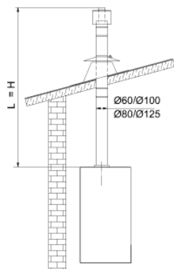
H = L Obrázek 3.8.2.1
