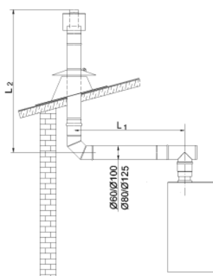
H = L_1 + L_2 + (1 \text{ m (ztráta na kolenu)}) + 1 \text{ m (ztráta na T-kusu)} Obrázek 3.8.2.2
