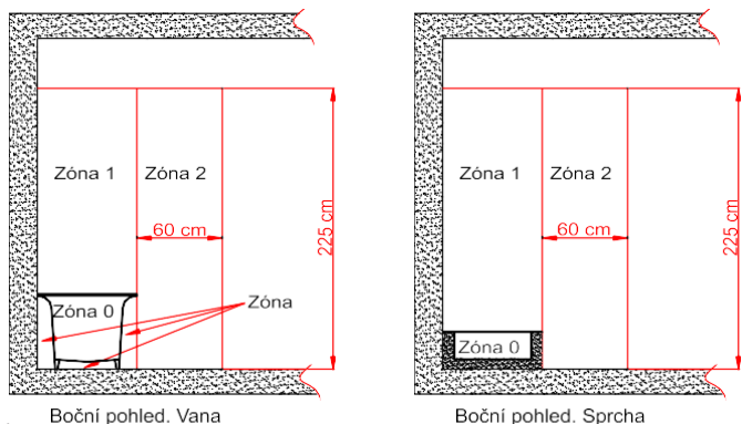
Obrázek 3.1.2.1 Rozměry zón v místnostech s vanou nebo se sprchou s bazénkem
