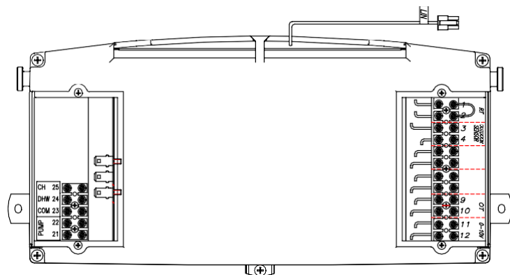
Obrázek 3.9.1.a Elektrické svorky řídicí jednotky pro dvoufunkční kotle
