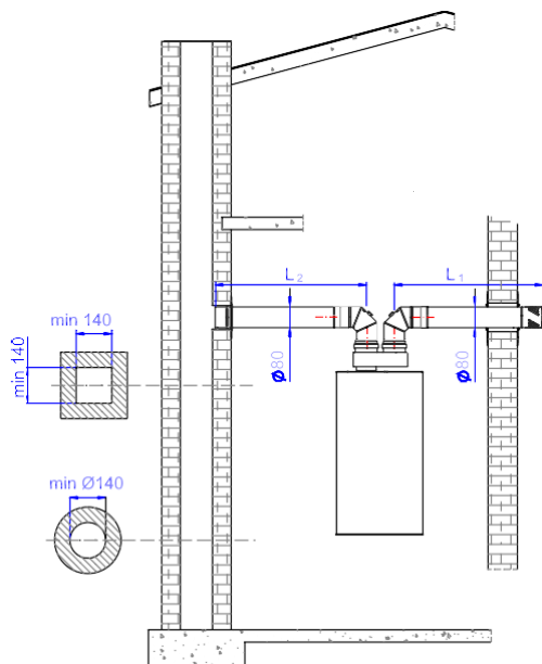
H = L_1 + L_2 + (1 \text{ m} + 1 \text{ m}) \text{ (ztráta na kolenech)} Obrázek 3.8.4.1
