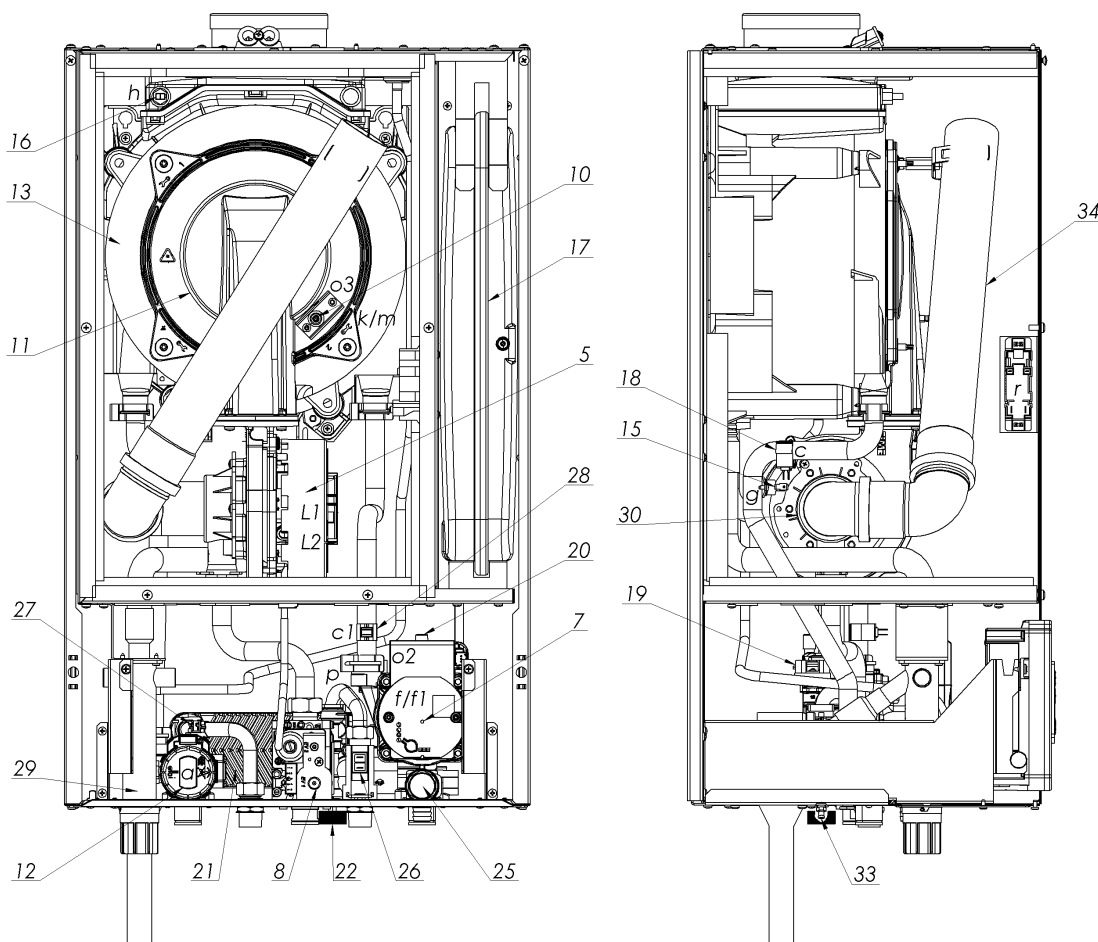
Obrázek 2.2.1.1 Uspořádání součástí ve dvoufunkčním kotli Ecocondens Nex
